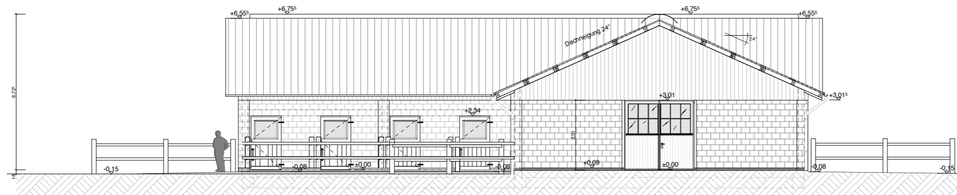
südansicht
