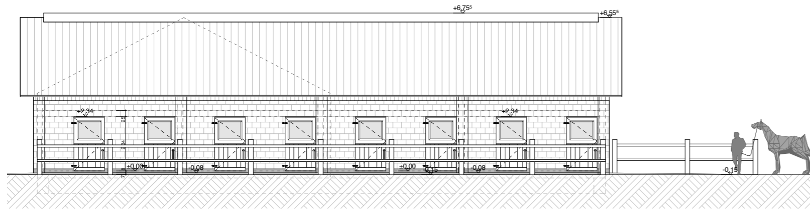
nordansicht
